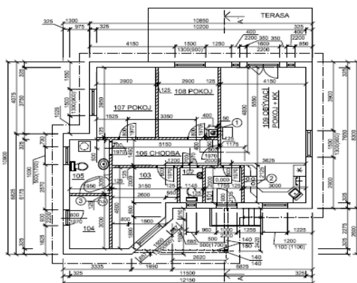
Obr. 1 – půdorys 1.NP
