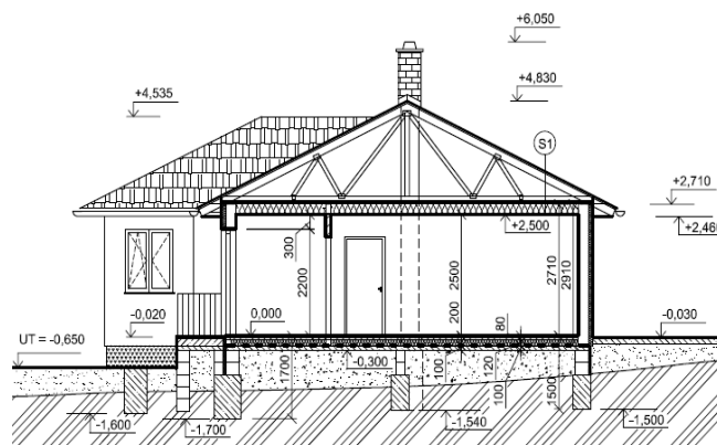
Obr. 2 – řez
