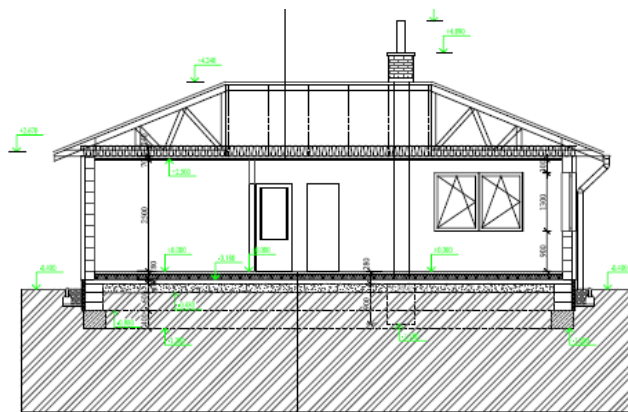
Obr. 2 – řez
