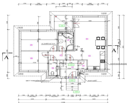
Obr. 1 – půdorys 1.NP
