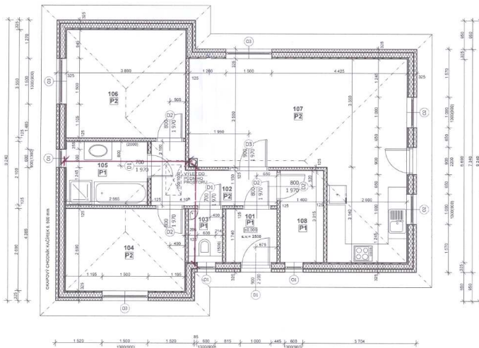
Obr. 1 – Půdorys 1.NP
