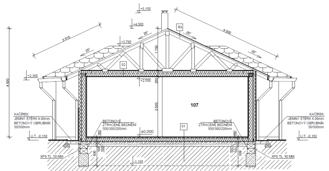
Obr. 2 – Svislý řez
