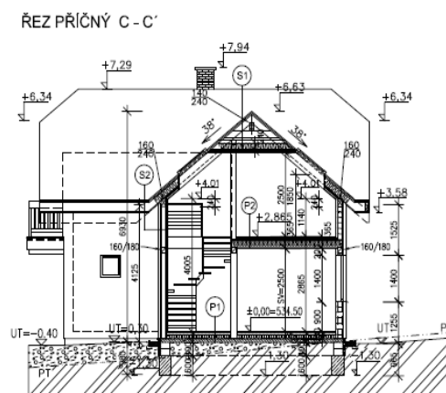
Obr. 2 – řez
