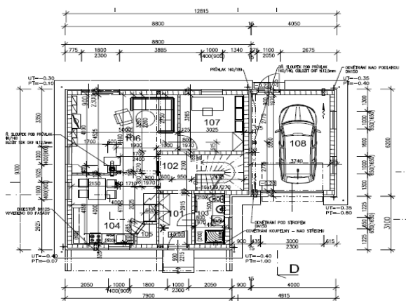
Obr. 1 – půdorys 1.NP
