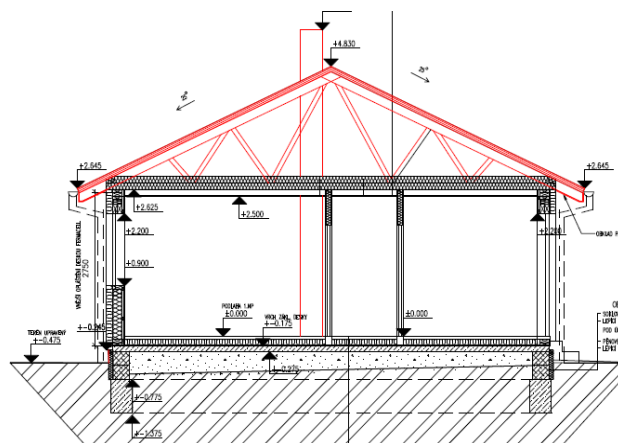
Obr. 2 – řez
